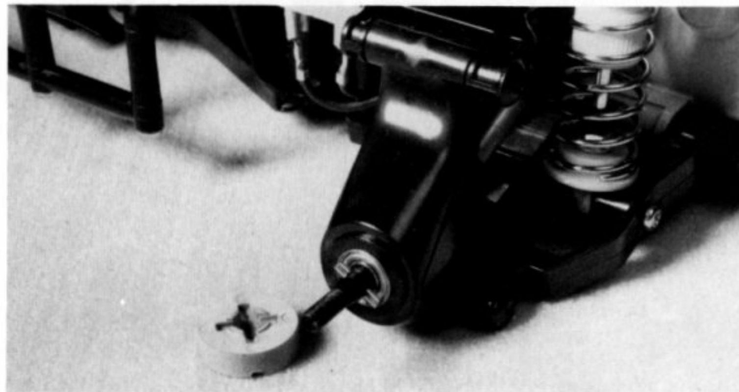
10. Bloquez les goupilles au moyen d'une petite goutte de colle anaérobie en prenant soin de ne pas en mettre sur le roulement. Ainsi vous ne risquez plus de les perdre en démontant les roues.
