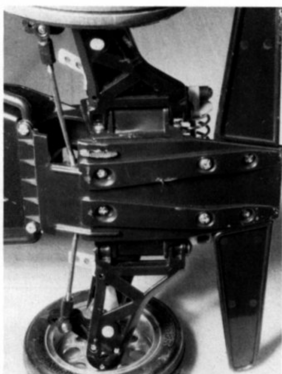
16. Le dessous de la coque est très bien protégé, ce qui est primordial en tout terrain. Mais ne serrez pas exagérément les vis.
