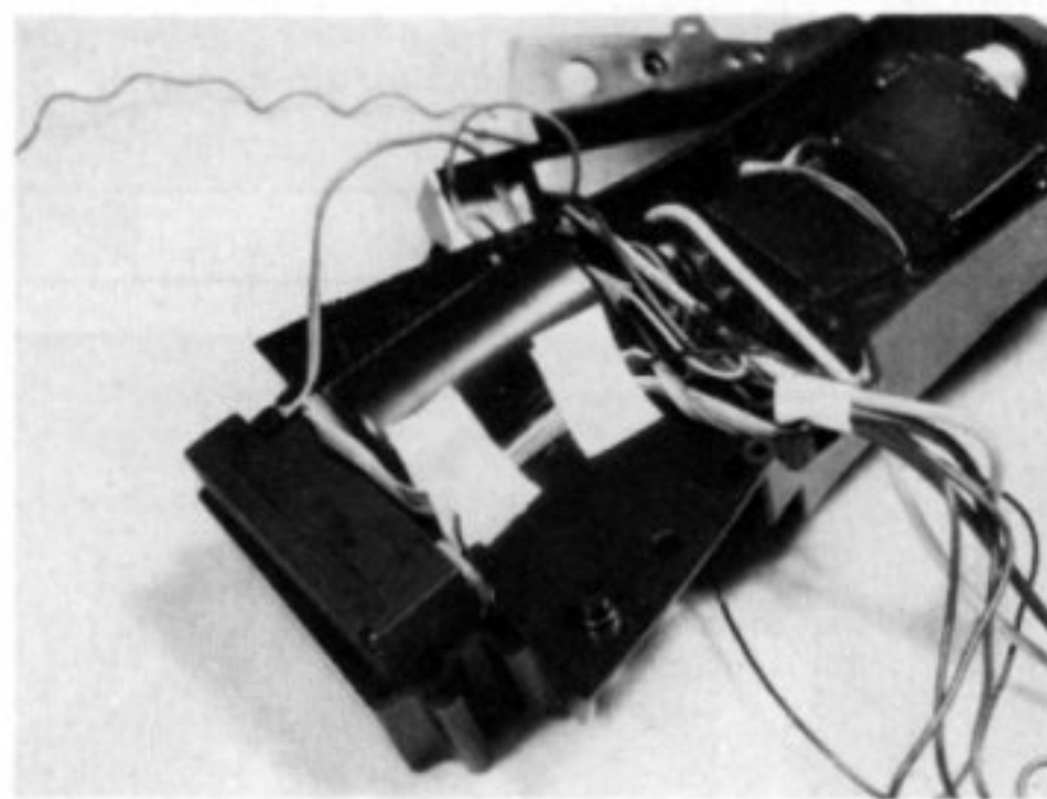
4. Avant de refermer la coque, soignez le guidage des fils car la place est comptée. Un peu de ruban adhésif permet de les maintenir en place.
