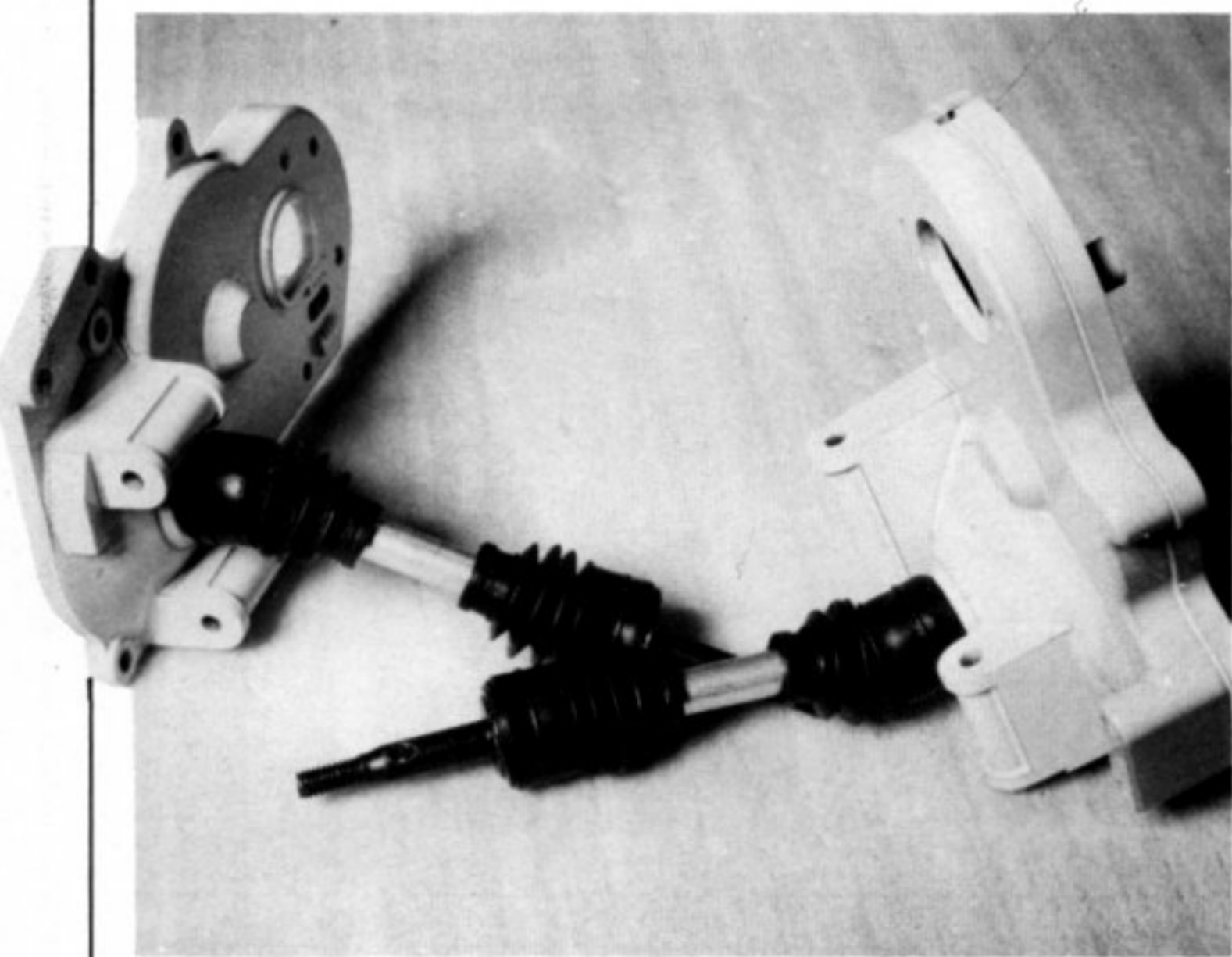
7. Vérifiez le graissage des cardans ; ne perdez pas les circlips de blocage des arbres d'entraînement à l'intérieur du carter !
