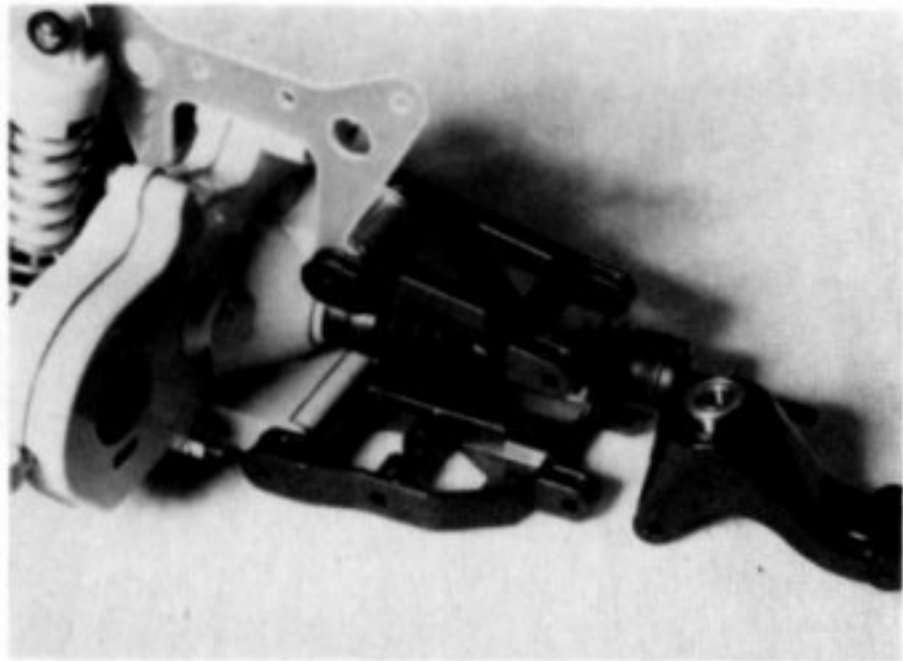
9. Le bloc arrière en cours de montage. Graissez bien les articulations et vérifiez le bon alignement des roulements à billes.
