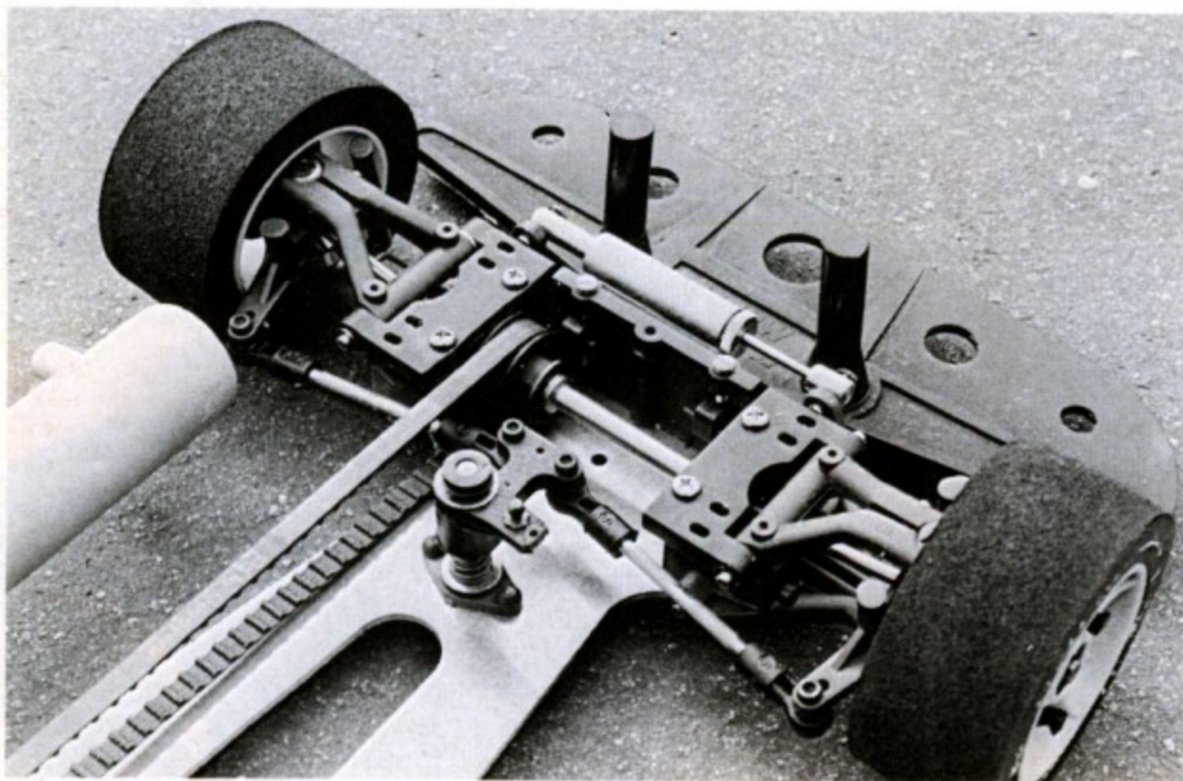
Le train avant dispose d'une multitude de réglage dont celui du carrossage. En plus toute la suspension est greffée sur le châssis.
