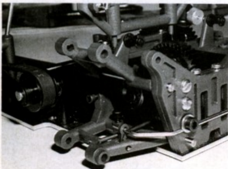
La barre anti-roulis est ancrée d'une manière mécanique. On distingue les vis de réglage des butées hautes et basses.
