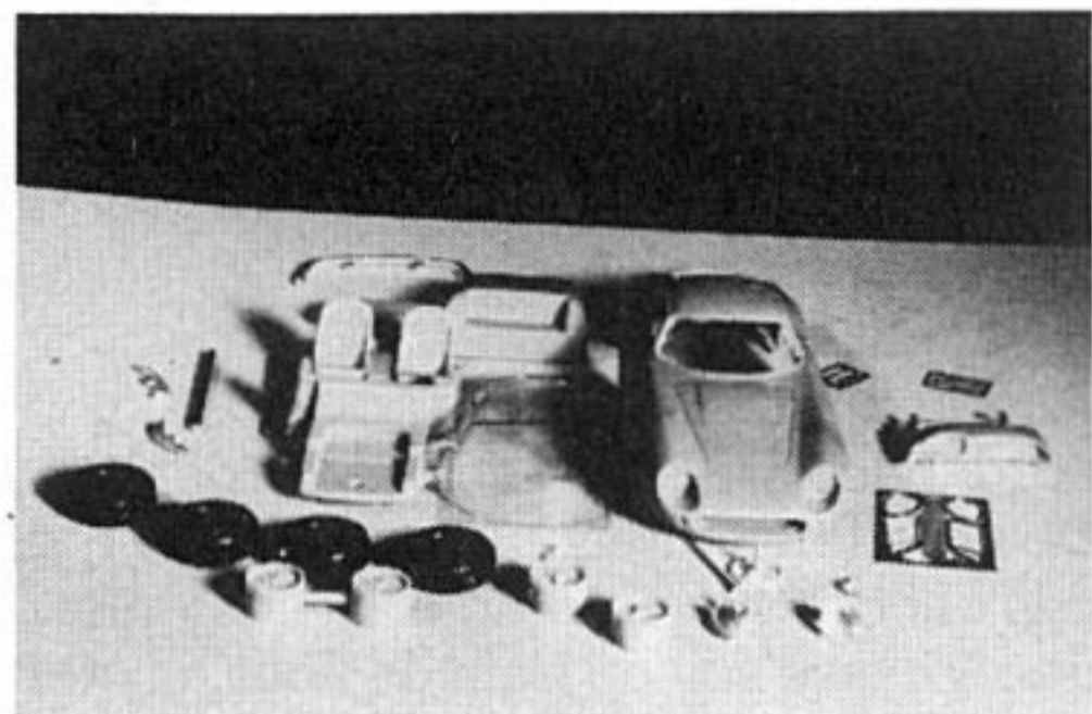
Ferrari 275 GTB 2 Provence Moulage.
