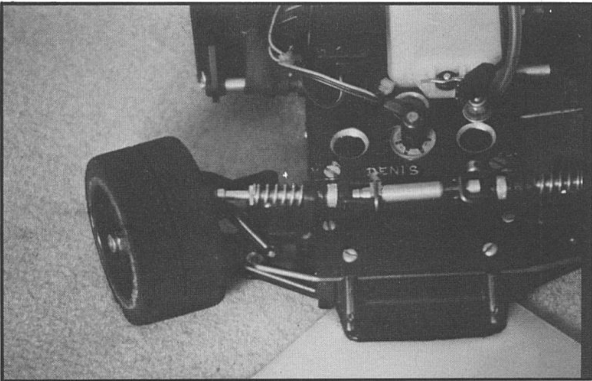
Les ressorts plus fermes de M. Torrès.
