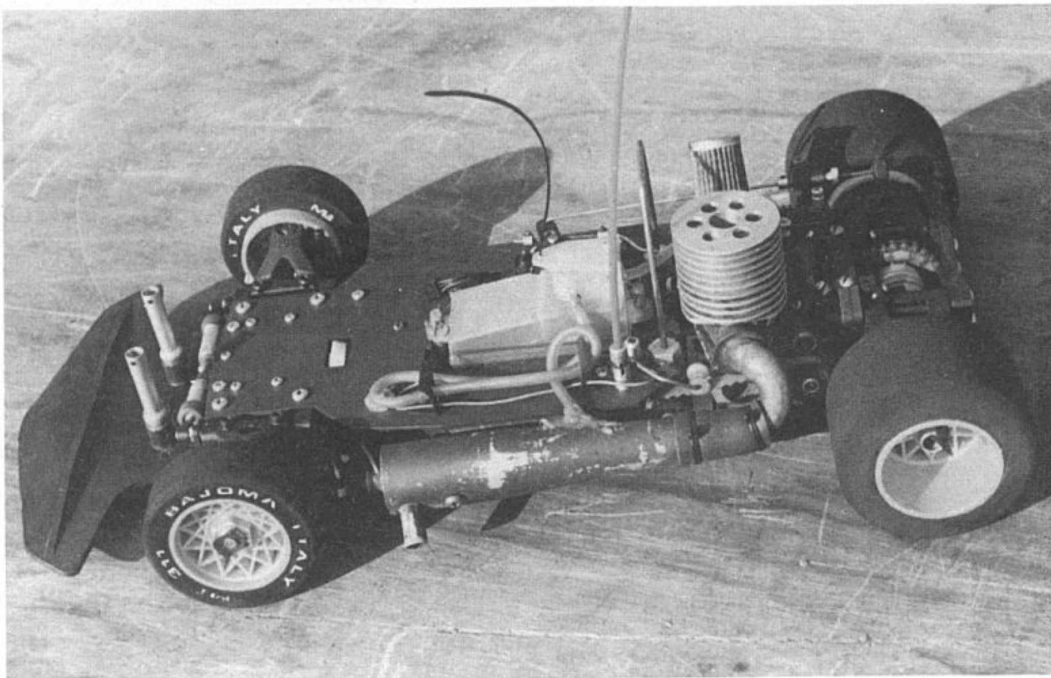
Serpent Quattro 4 WD
