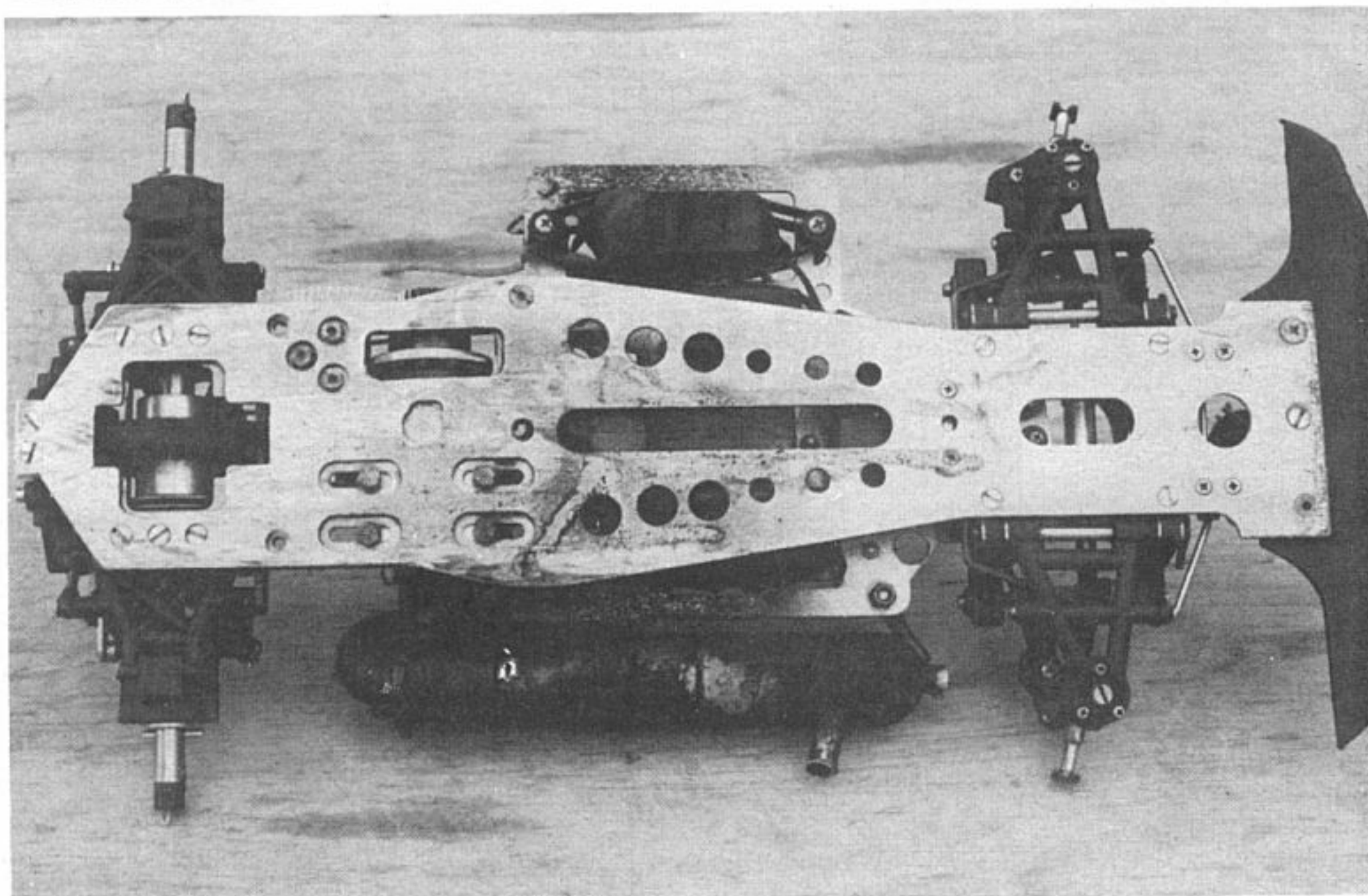
SG Columbia MK IV
