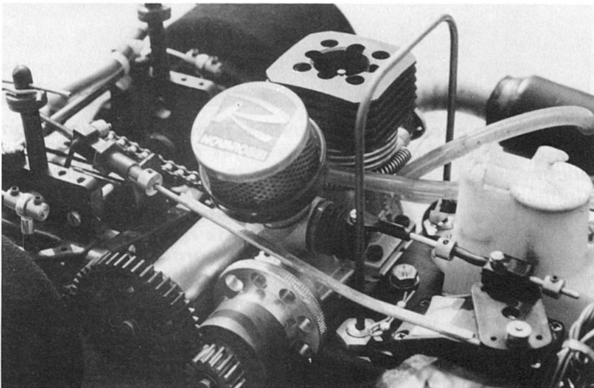
Le Nova Rossi Testa Rossa
