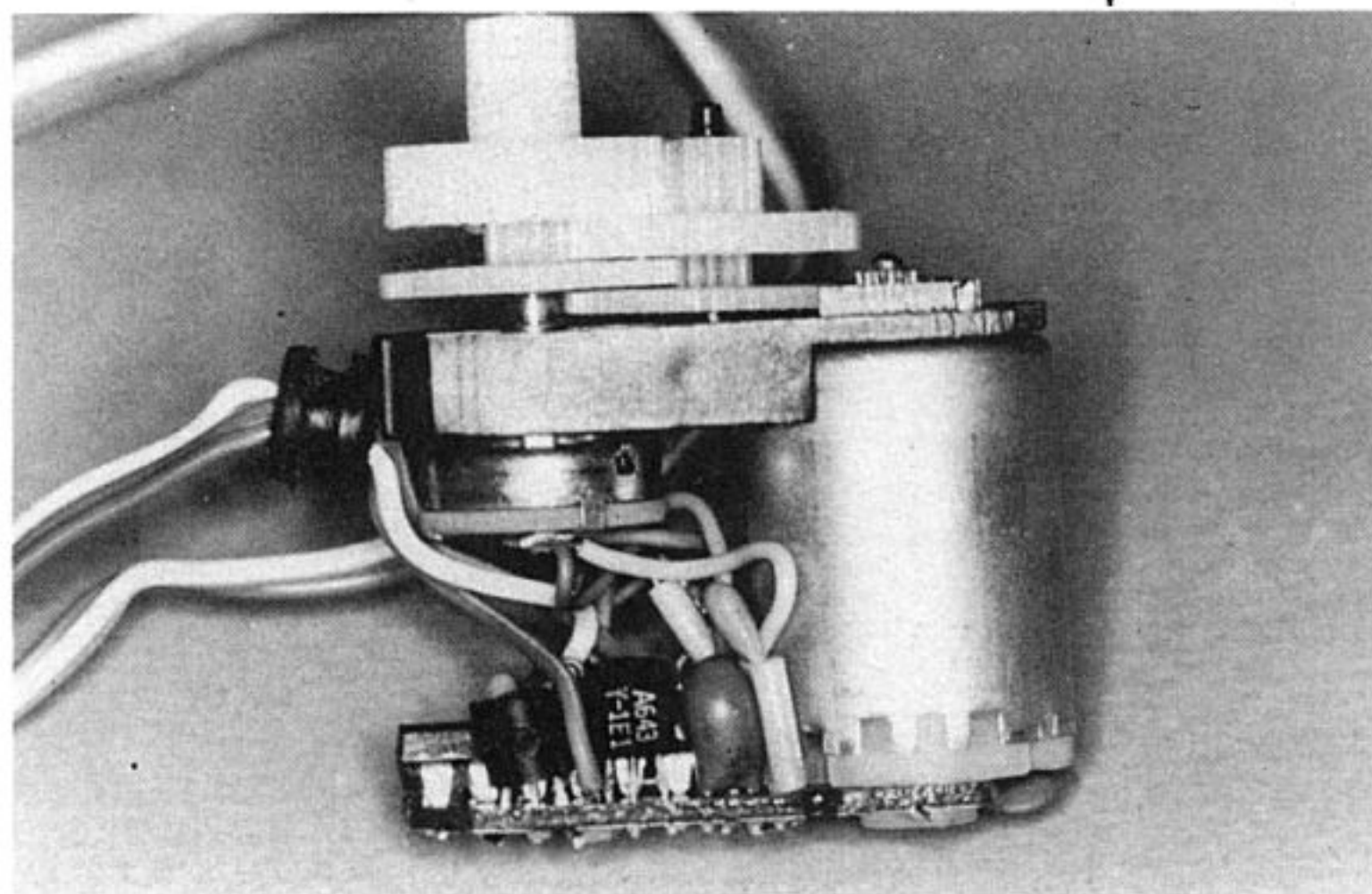
Le potentiometre est solidaire de l'axe de sortie
