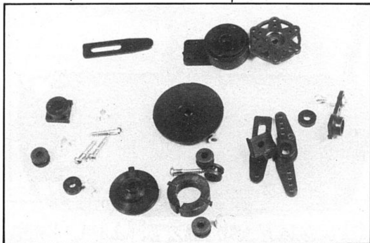
Divers types de palonniers, dont un réglable
