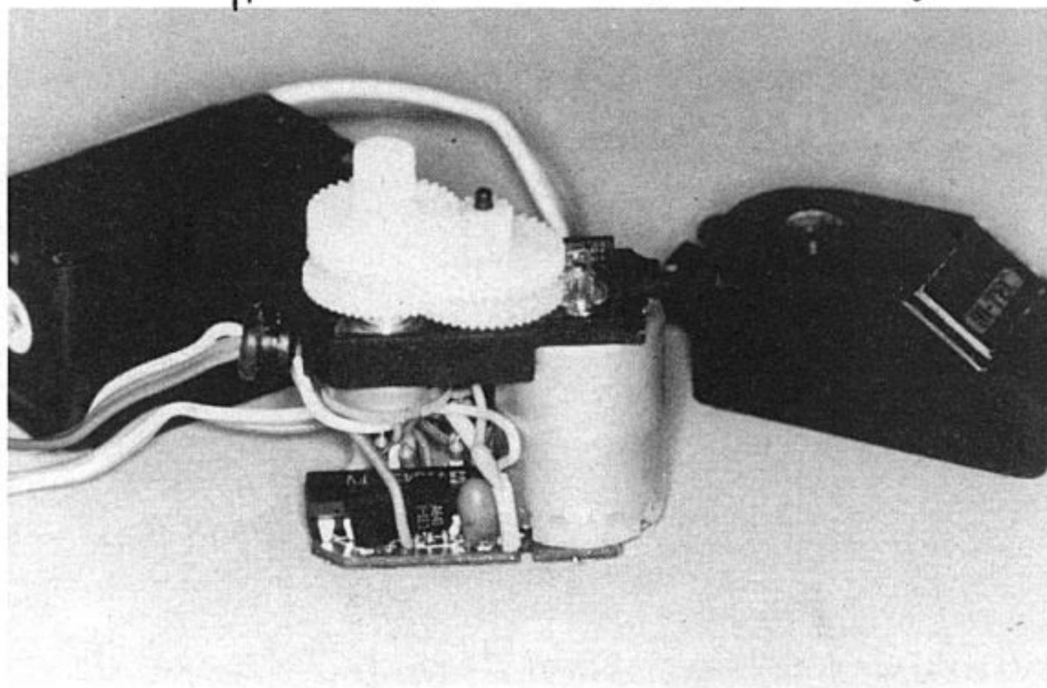
La pignonnerie du reducteur est en plastique
