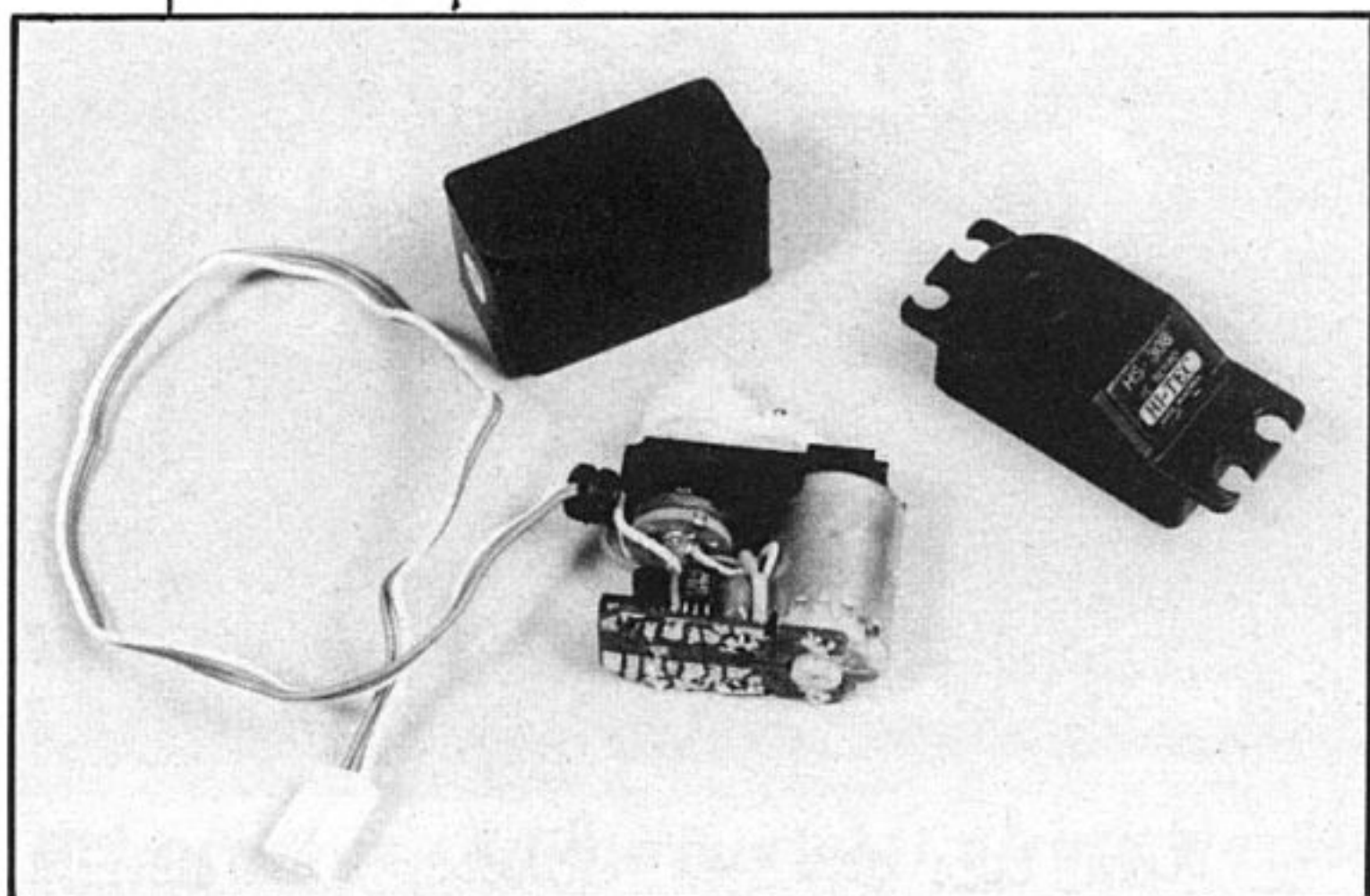
Le boitier de servo est en deux parties
