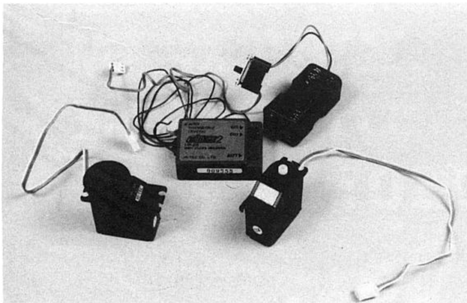
La partie reception avec ses deux servos
