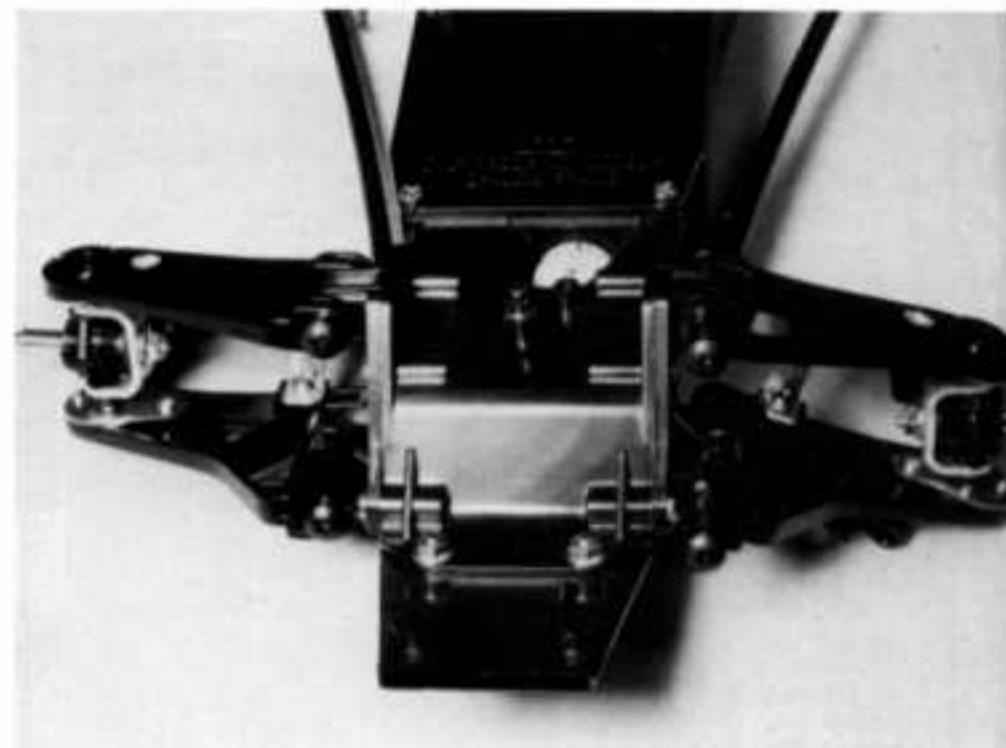
12. Le train avant comporte un mélange de pièces plastiques et métalliques. Ne serrez pas trop les vis afin de ne pas endommager les filets qui se forment au fur et à mesure.
