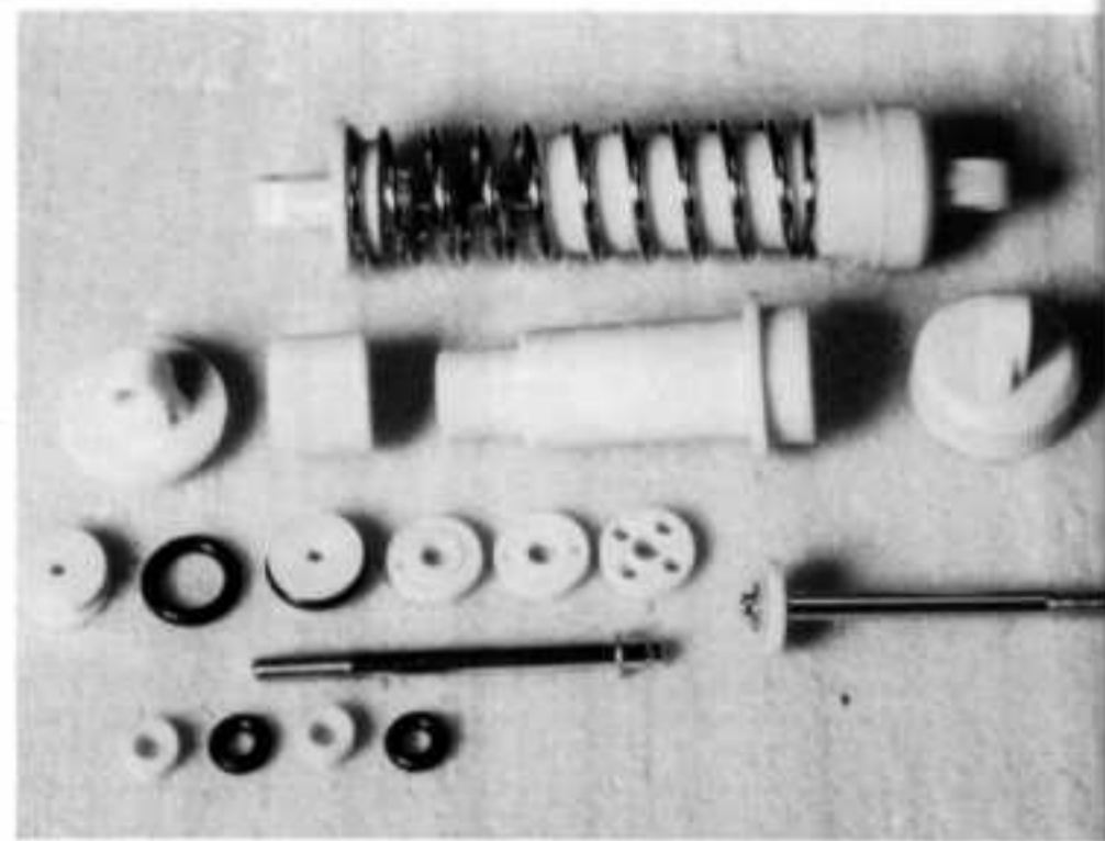
8. Voici comment se présentent les amortisseurs. Trois pistons, percés ou non, permettent de faire varier le flux d'huile et complètent les possibilités de variation d'amortissement obtenue habituellement par le seul changement de viscosité.
