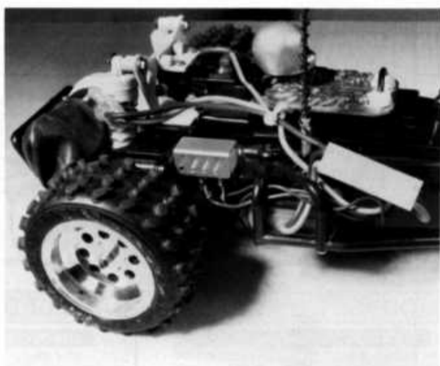
18. Pour terminer, protégez les ouvertures du moteur au moyen du ballon de baudruche dont vous coupez le goulot et guidez bien les fils d'alimentation afin qu'ils ne touchent pas les articulations ni les résistances.
