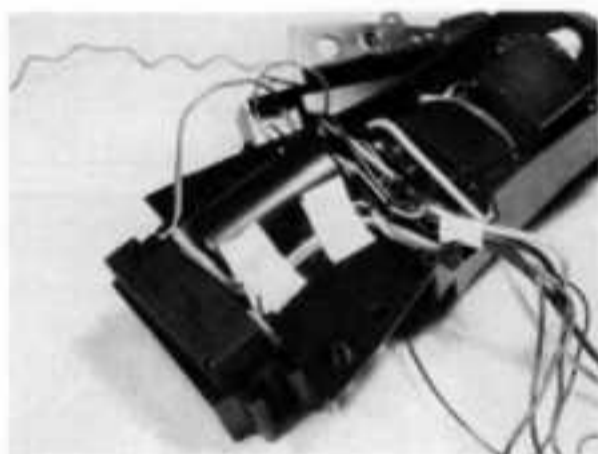
4. Avant de refermer la coque, soignez le guidage des fils car la place est comptée. Un peu de ruban adhésif permet de les maintenir en place.
