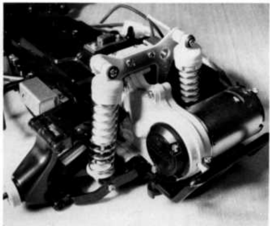
11. Le train arrière est maintenant entièrement monté et le moteur est installé. Remarquez en haut des amortisseurs la bague réglant la dureté des ressorts.
