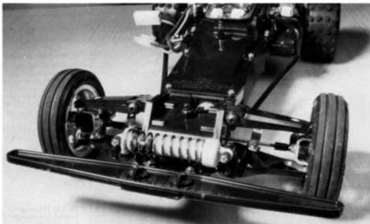
15. On voit bien ici le montage de l'amortisseur avant (sans bague) et du pare-chocs. Réglez les tringles pour obtenir un pincement des roues de 3°, amortisseur au repos.
