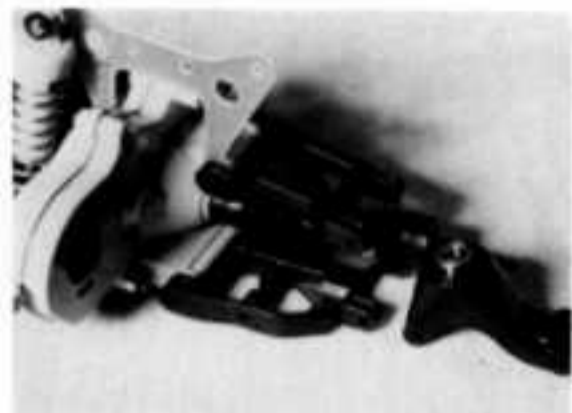
9. Le bloc arrière en cours de montage. Graissez bien les articulations et vérifiez le bon alignement des roulements à billes.
