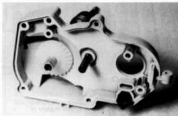
6. Soignez l'implantation des éléments dans le carter, ébarbez si nécessaire, vérifiez les jeux et graissez abondamment au bisulfure de molybdène au moyen du tube fourni.
