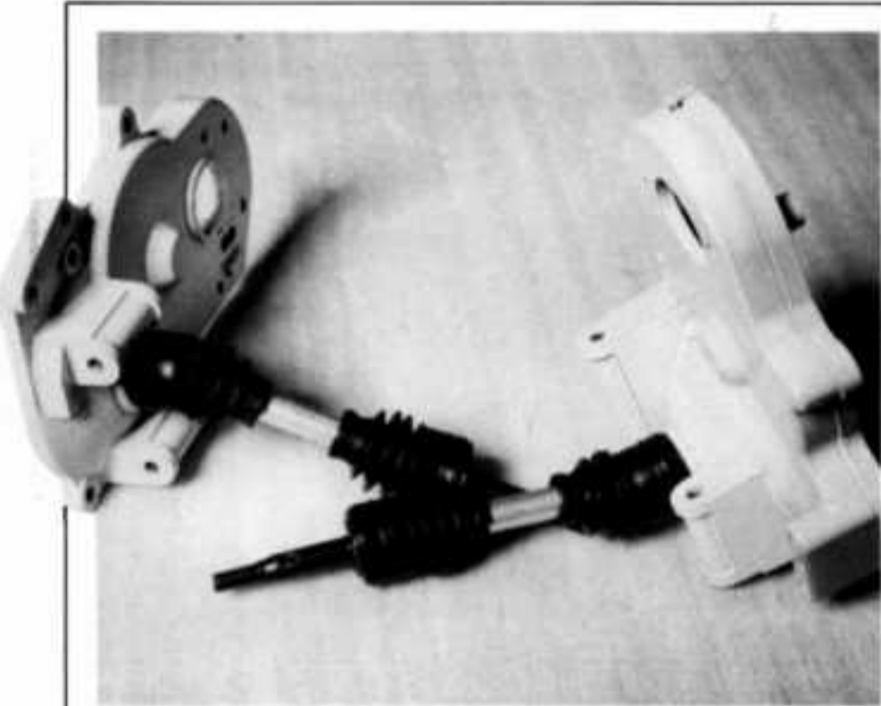
7. Vérifiez le graissage des cardans ; ne perdez pas les circlips de blocage des arbres d'entraînement à l'intérieur du carter !
