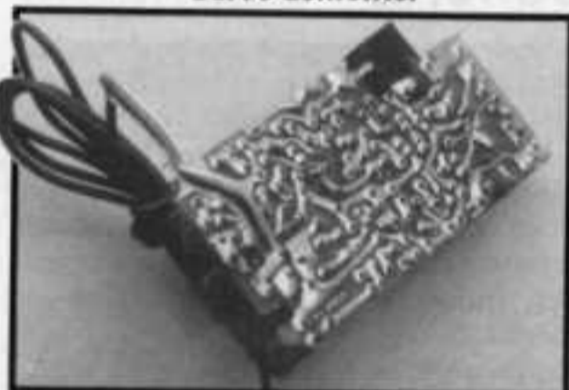
Servo démonté.
