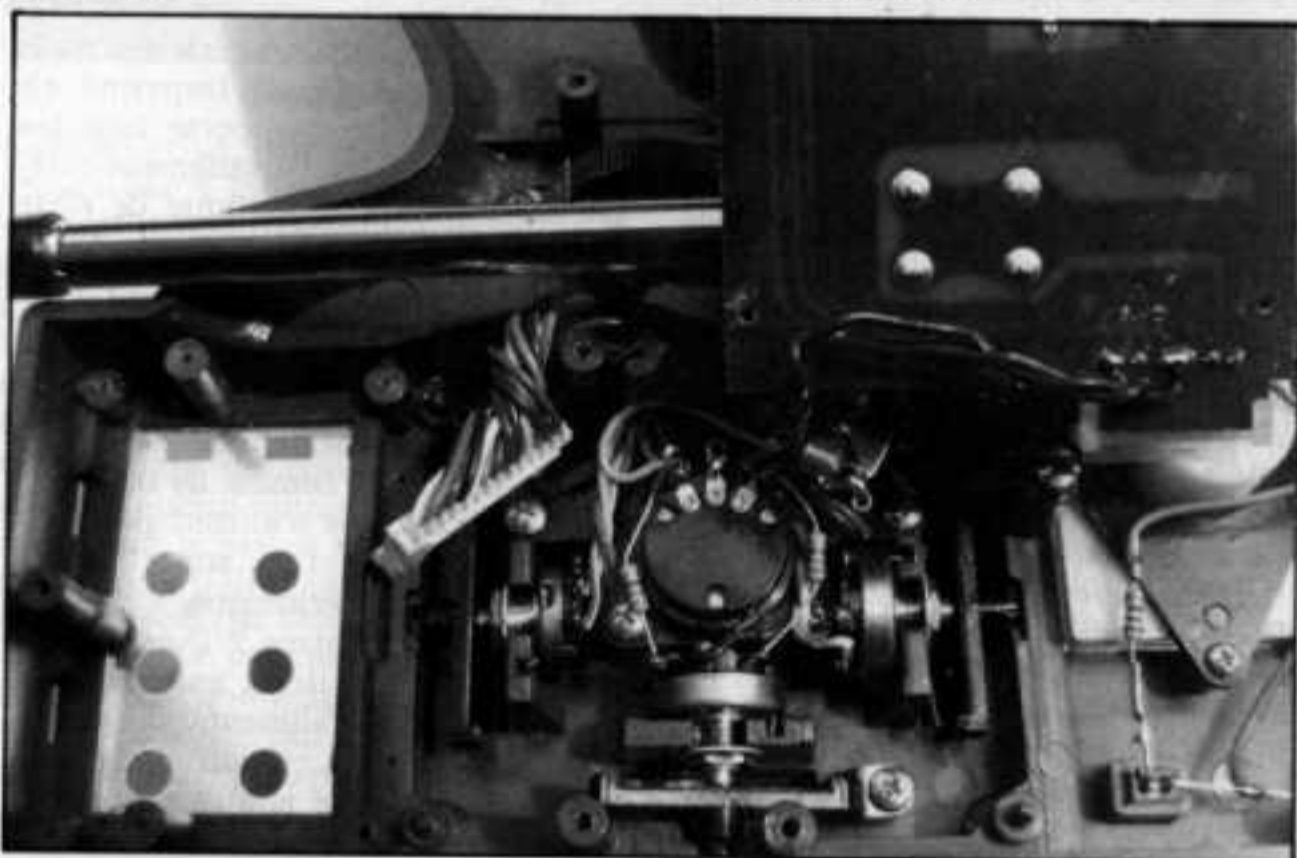
Commande des trims électroniques.
