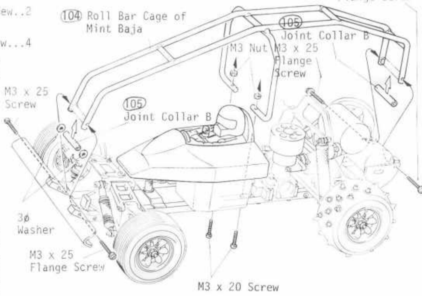
M3 x 25 Flange Screw
